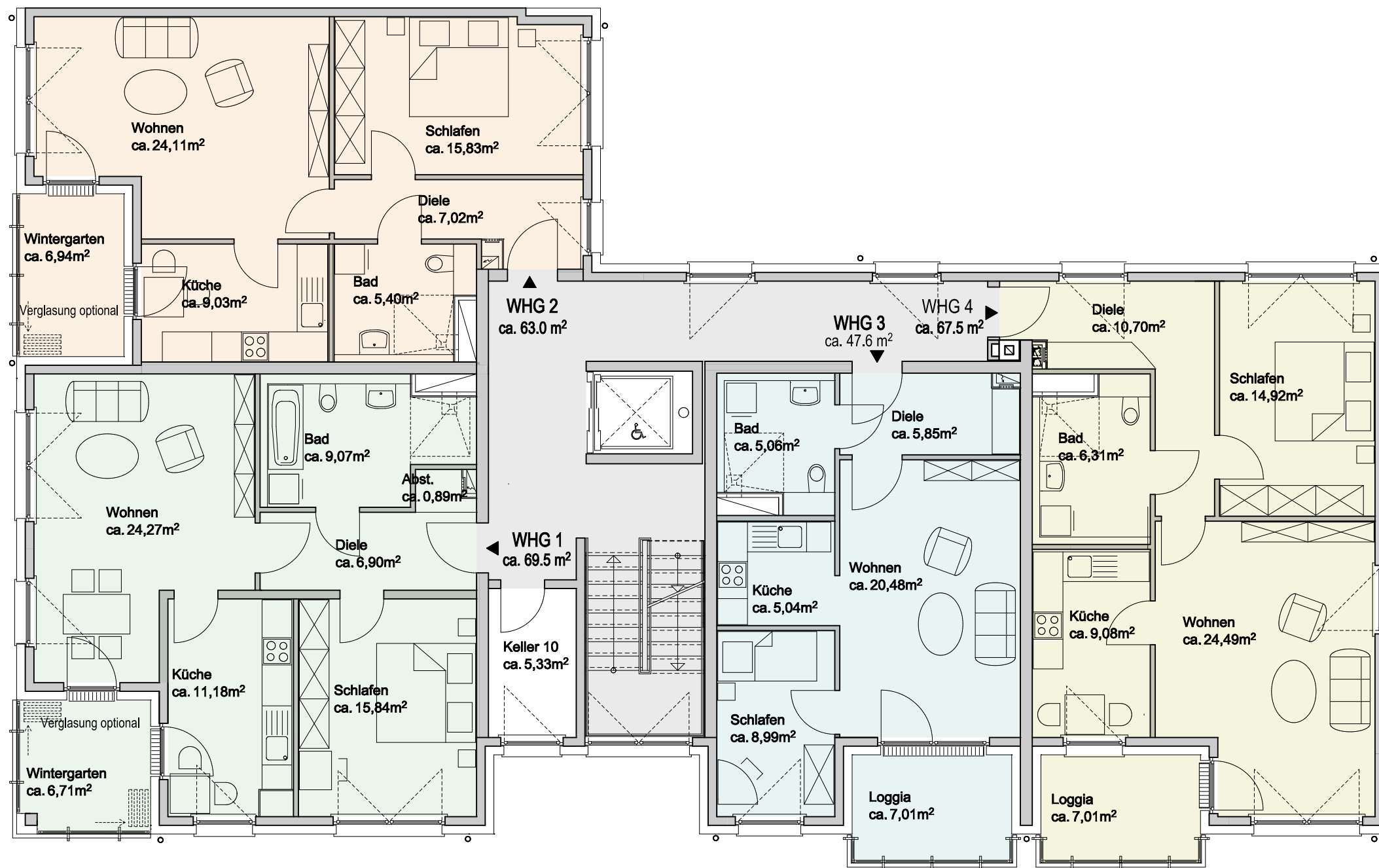
1. OBERGESCHOSS
